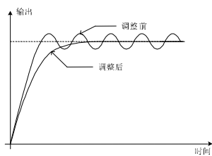
图 6-28 抑制输出周期振荡
