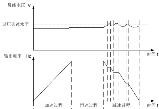
图 6-21 过压失速动作过程示意图
