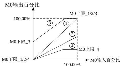
图 6-11 M0 输出百分比曲线图
