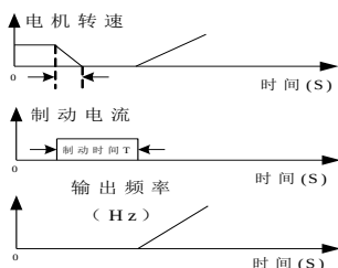
图 6-12 启动直流制动过程
