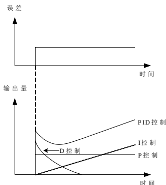
图 6-25 PID 控制的作用
