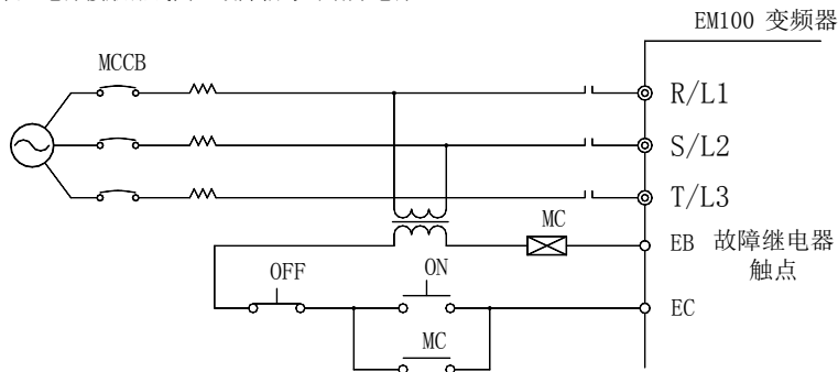
图 3-6 接入输入断路器
