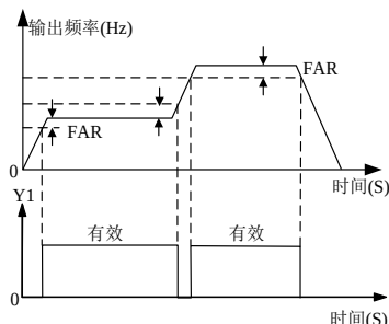
图 6-16 频率到达检测范围 FAR
