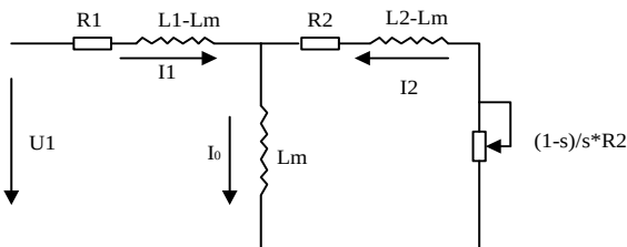
图 6-8 异步电动机稳态等效模型
