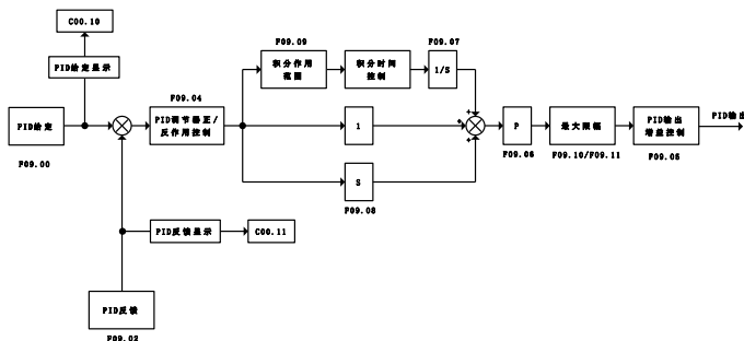
图 6-26 EM100 内部过程 PID 的控制逻辑图
