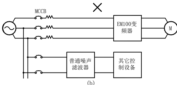
图 3-8 噪声滤波器的错误安装
