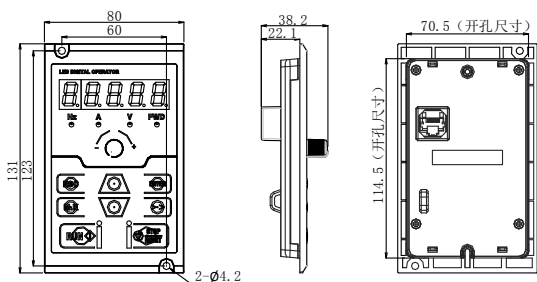
(d) A90-4T060KEY3 外引键盘外形
