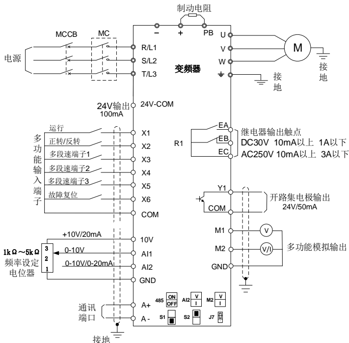
图 3-10 控制回路标准接线图
